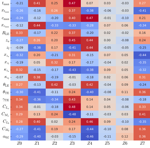
(a) Latent parameter traversal data
